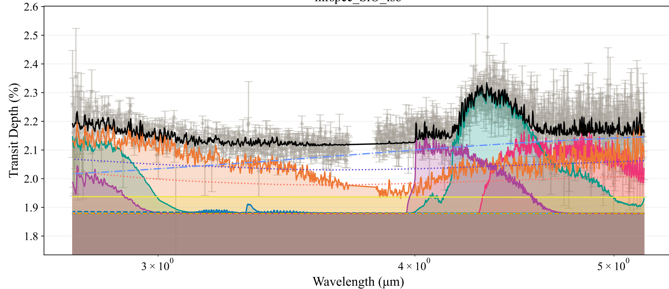
nirspec_SiO_iso
